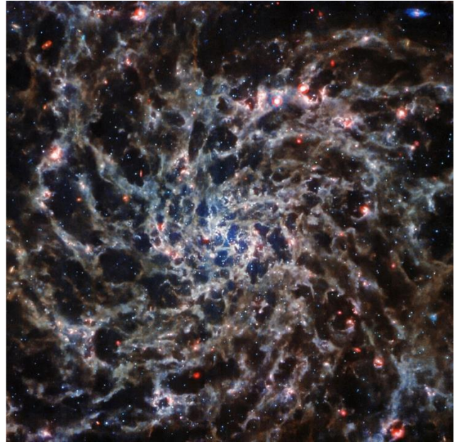
JWST の中間赤外線画像
